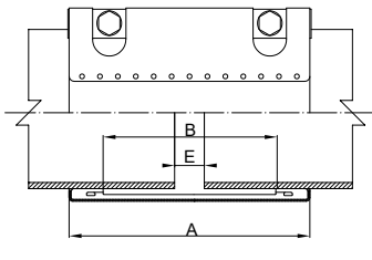
SECCIÓN TRANSVERSAL
